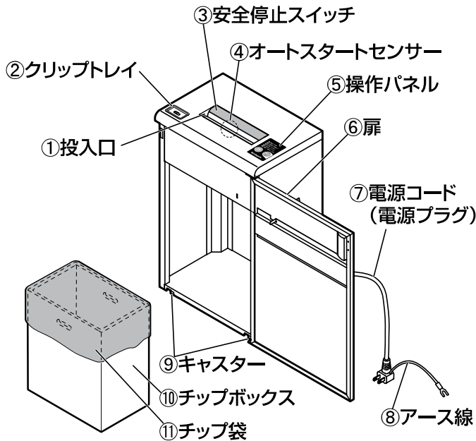
図1 外観図
