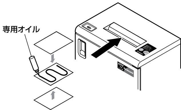
図5 注油方法
