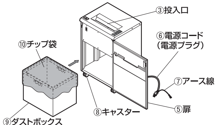
図6 ダストボックスのセット
