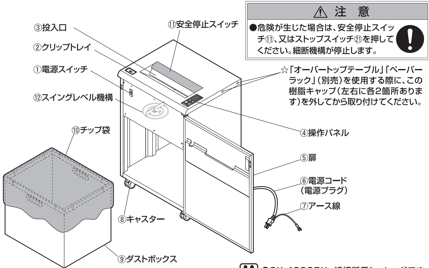
図1 外観図
