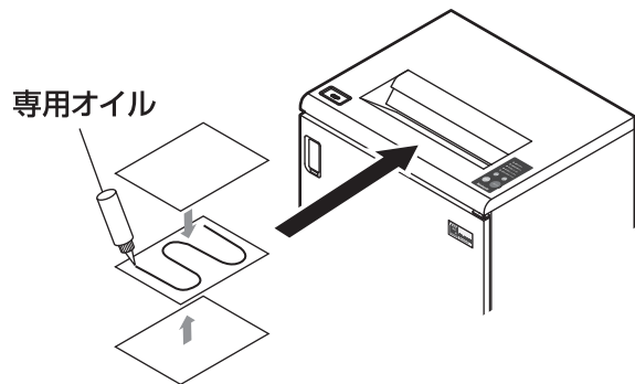
図9 注油方法
